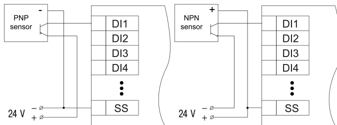
Fig. 6 PNP sensor wiring (MV210-202)
