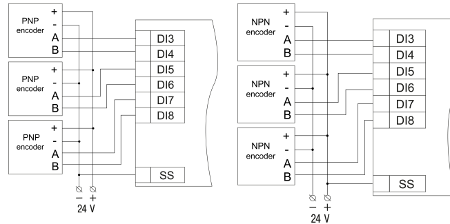
Fig. 9 PNP encoder wiring
