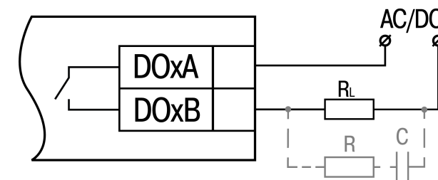
Fig. 3 Relay wiring
